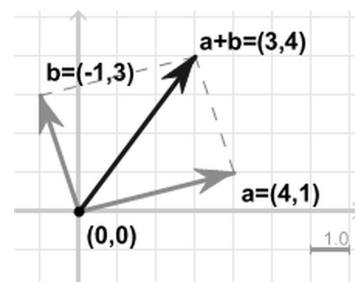
Slika 1.1: Veza prostora usmerenih duži u ravni i \mathbb{R}^2 .
