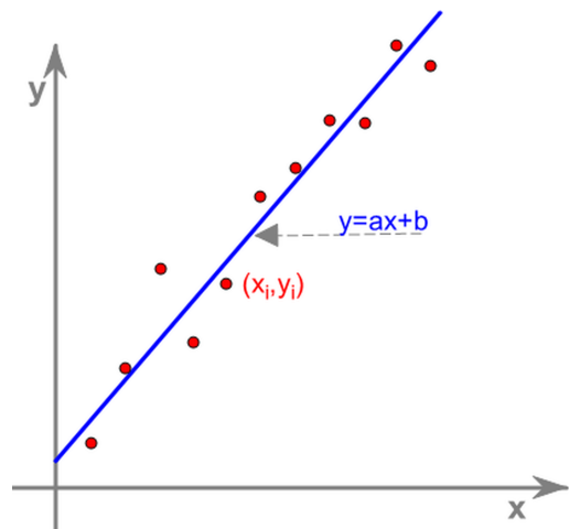
Slika 1.13: Grafički prikaz merenih veličina i fit prave linije.
