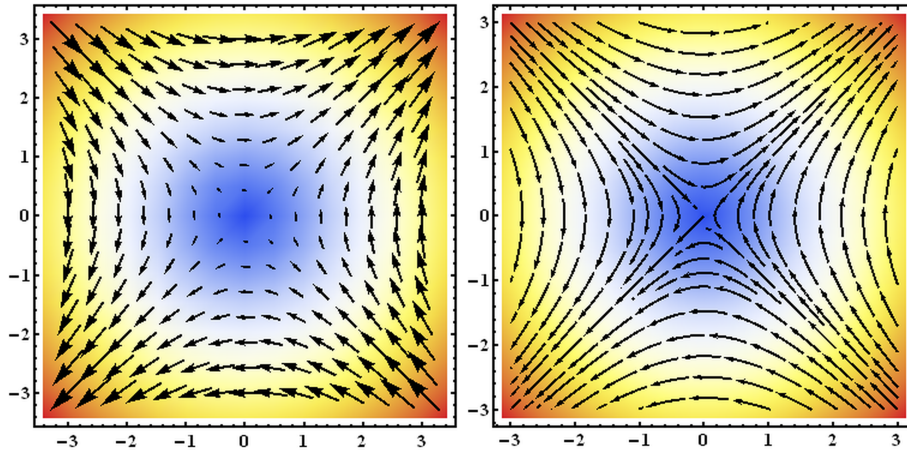
Slika 3.4: Prikaz vektorskog polja (u ravni) pomoć u vektora (levo) i strujnih linija (desno). Boja označava gustinu polja u datoj oblasti.
