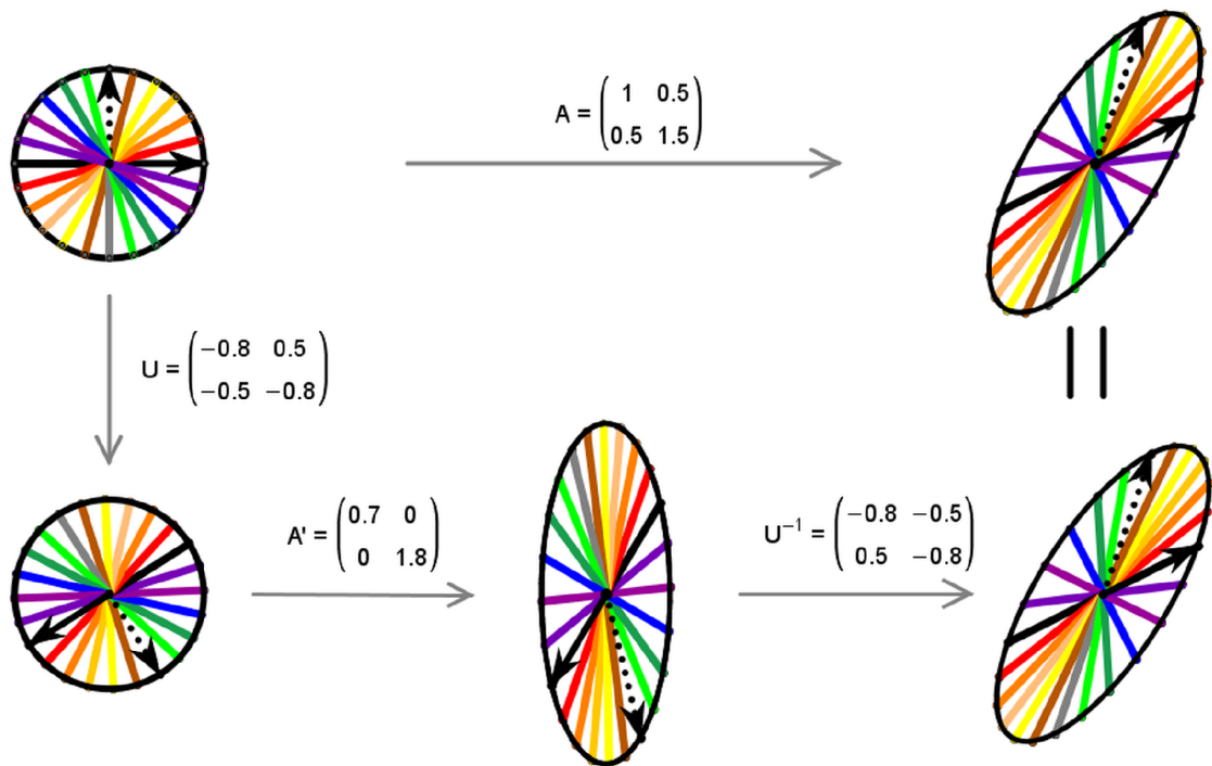
Slika 2.11: Unitarna sličnost matrice A .
