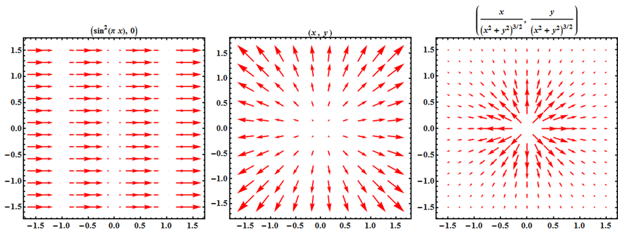
Slika 3.7: Primeri vektorskih polja u ravni (zadatak 3.3.1).
