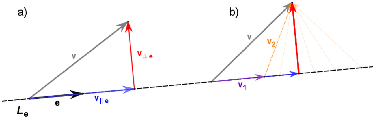
Slika 1.9: a) Projekcija i normala vektora \mathbf{v} na pravac L_{\mathbf{e}} . b) Slika uz Primer 1.2.9.
