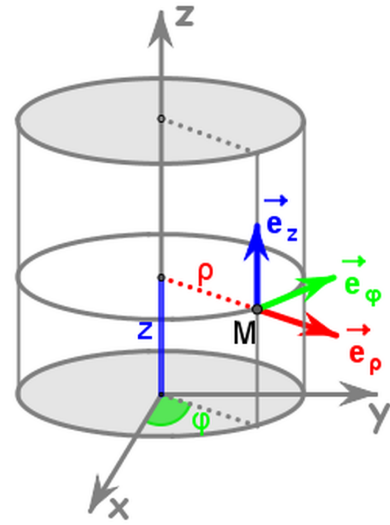
Slika 3.12: Cilindrični koordinatni sistem.
