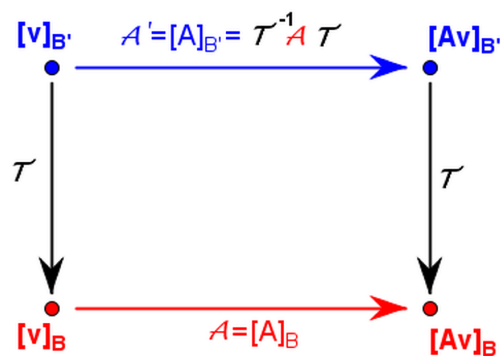
Slika 2.7: Dijagram promene bazisa.
