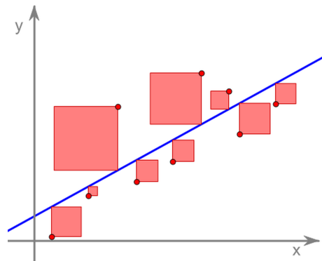
Slika 1.14: Interpretacija MNK preko minimiziranog zbira površina.
