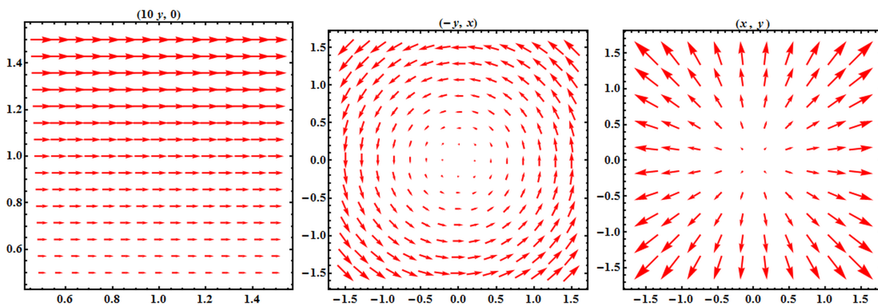
Slika 3.10: Primeri vektorskih polja u ravni (zadatak 3.4.1).
