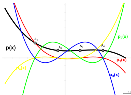
Slika 1.5: Interpolacioni polinom za tačke A_1, A_2, A_3, A_4 .
