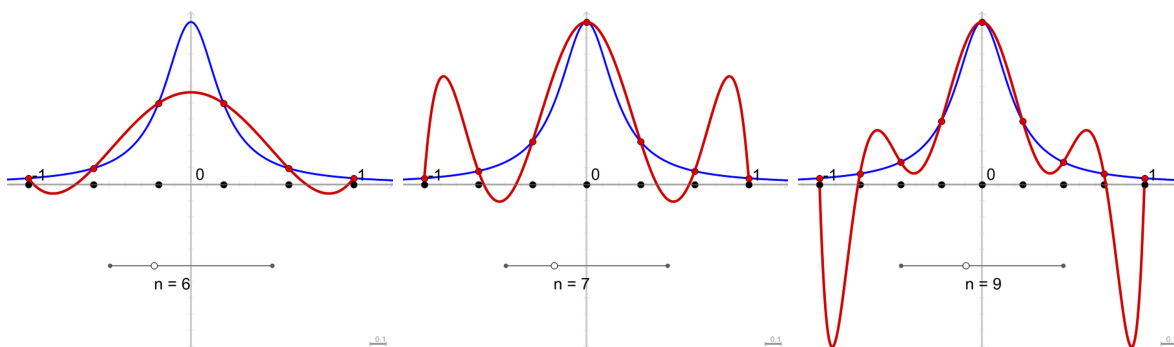
Slika 1.6: Grafik funkcije f(x) = 1/(1 + 25x^2) (plavo) i grafici interpolacionih polinoma (crveno) stepena 5 (levo), 6 (u sredini) i 8 (desno).
