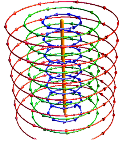
Slika 3.5: Vektorske linije magnetnog polja oko pravolinijskog provodnika.
