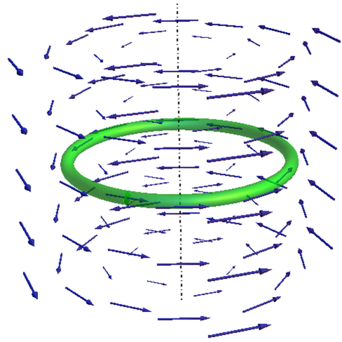
Slika 3.8: Tanko crevo potopljeno u tekući fluid.
