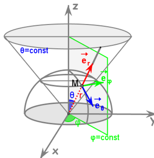
Slika 3.13: Sferni koordinatni sistem.
